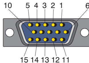
Stecker von Lötseite gesehen
